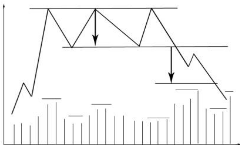
图 6-43 三重顶
