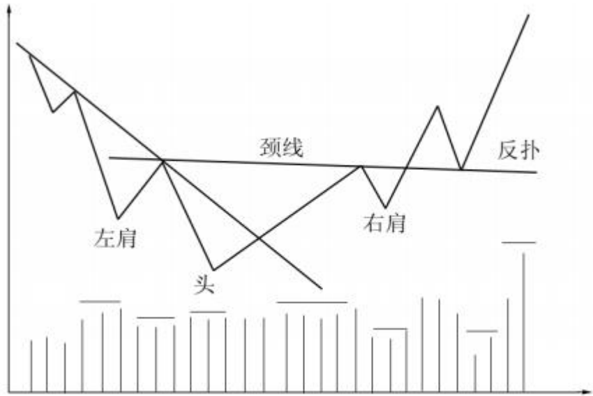
图 6-41 头肩底形态
