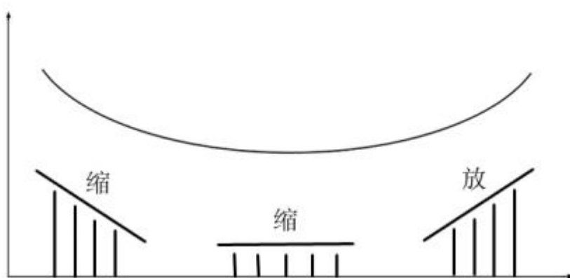
图 6-44 圆弧底
