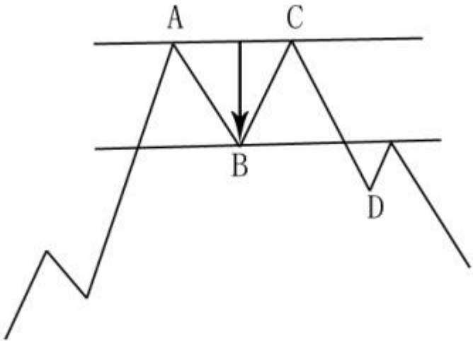
图 6-42 双重顶（底）
